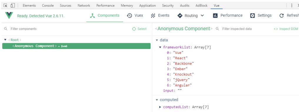
Figure 3.35: Chrome extension for Vue.js DevTools
